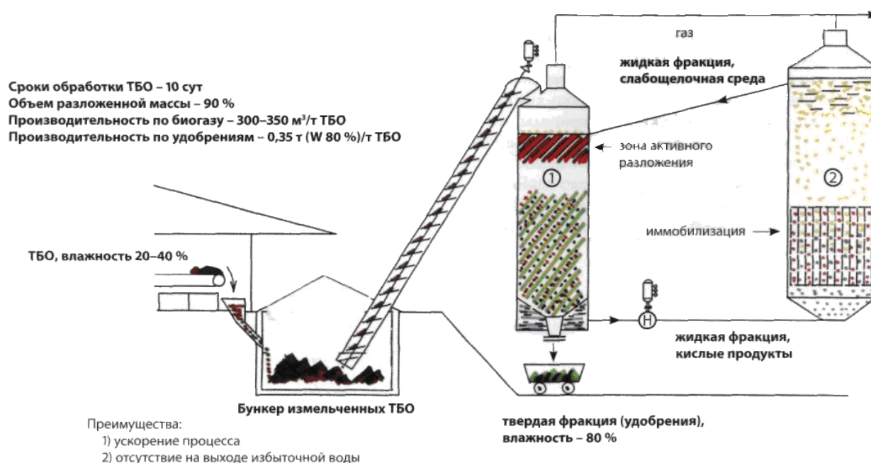
Рисунок 2. Схема рециркуляционно-твердофазной термофильной биометангенерации (разработано автором)
