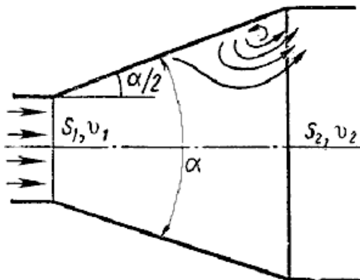
Рисунок 4. Постепенное расширение трубы
