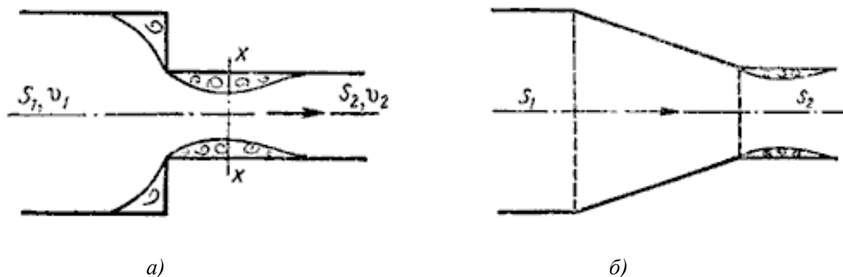
Рисунок 2. Сужение трубы: а-внезапные, б-постепенные
