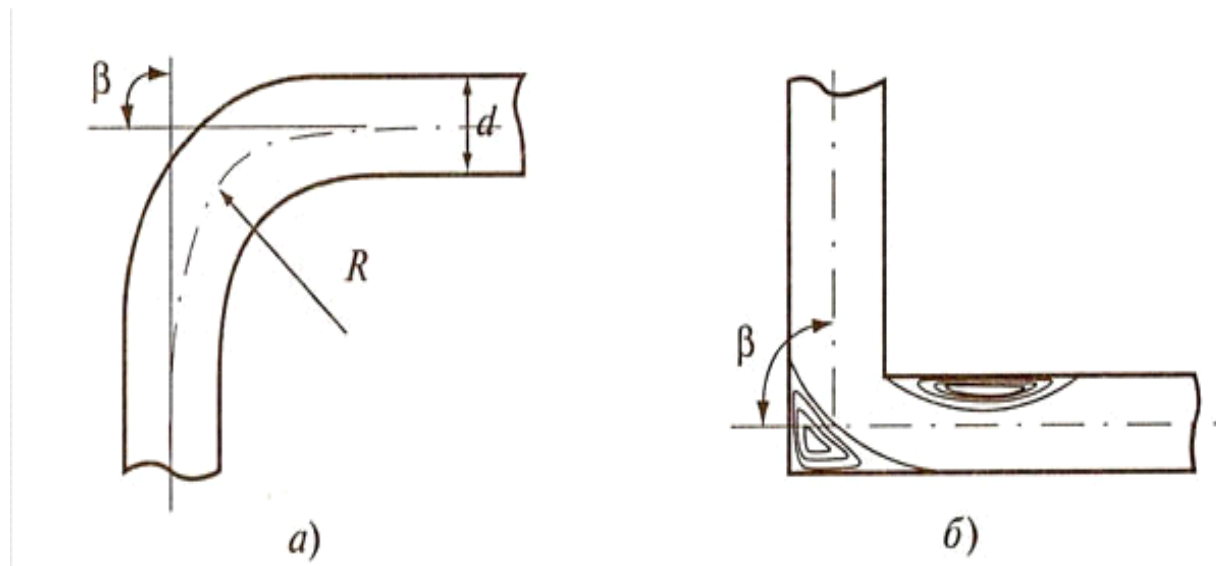
Рисунок 1. Виды местных сопротивлений в трубопроводах
