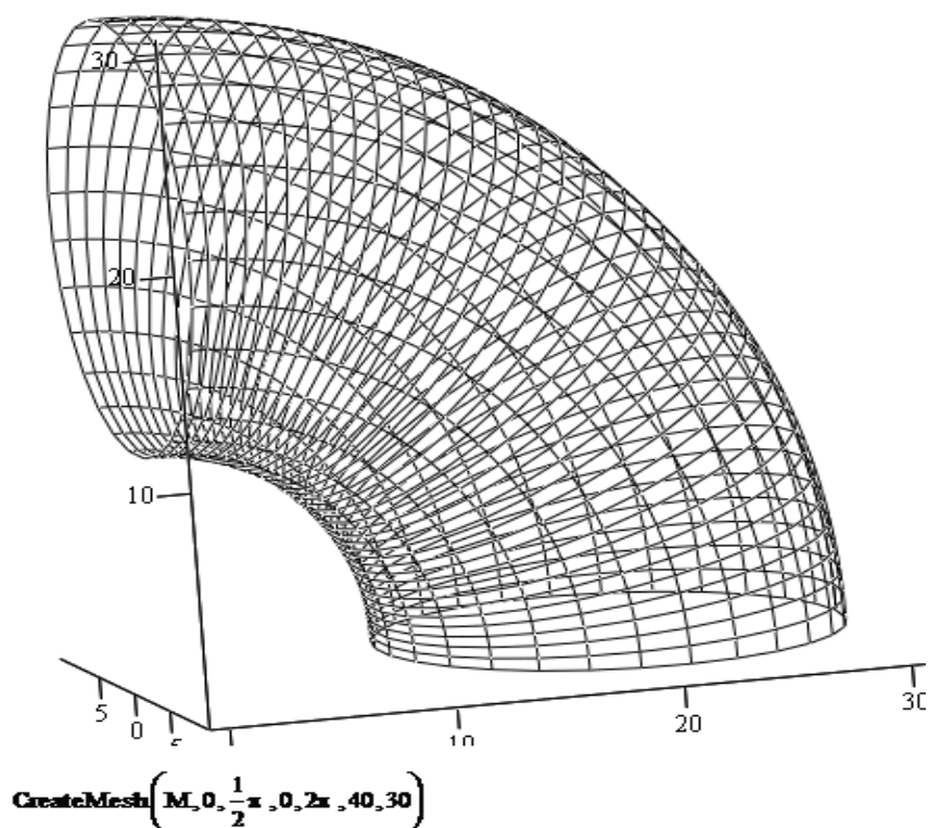
Рисунок 5. Моделирование дугового колена трубы по аналитическим зависимостям
