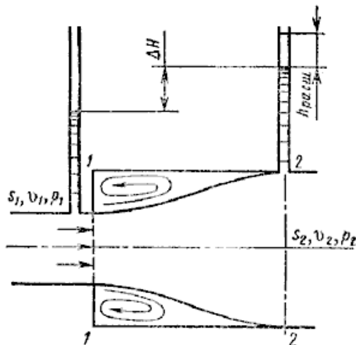
Рисунок 3. Внезапное расширение трубы
