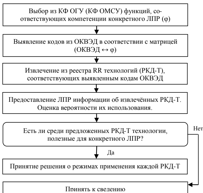
Рисунок 2. Схема функционирования процедур предоставления информации о РКД-Т для ЛПП
